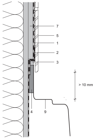
Abb. 6.4-2 Beispiel: Anschluss Duschtasse – Wand mit hochgezogenem Duschtassenrand
