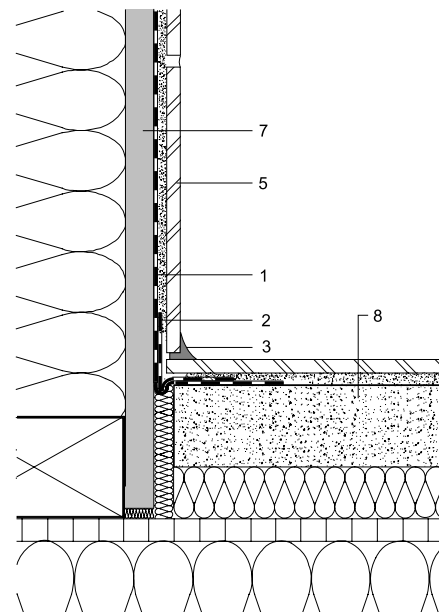
Abb. 6.3-3 Beispiel: Boden-Wand-Anschluss
